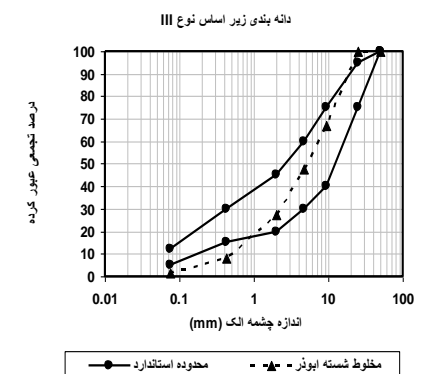
شکل ۲ نتایج آزمون مخلوط شکسته یکی از کارگاه‌های استان خراسان شمالی
