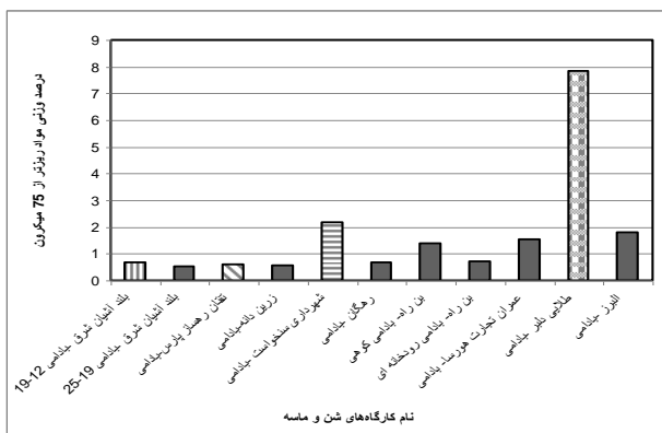
شکل ۵ نمودار ستونی مواد ریزتر از ۷۵ میکرون در شن بادامی کارگاه‌های استان خراسان شمالی
